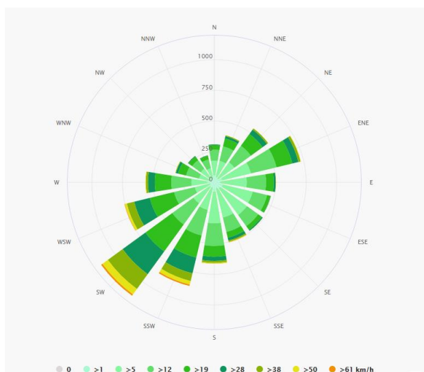
Рис. 1. Роза ветров
