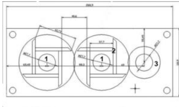
Рис.6. Креслення двухвалового подрібнювача: 1 вали, 2 – ніж, 3 – приводний шестерня
