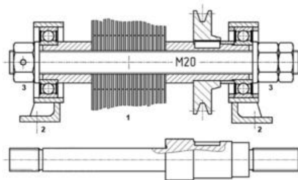
Рис.4. Креслення подрібнювача з дискових пилок: 1 – комплект пив до 20 шт. товщиною 6-10 мм, 2 – місця кріплення на раму, 3 – гайки-фіксатори.
