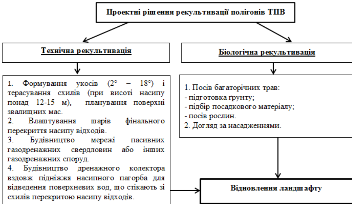
Рис. 1. Схема технології рекультивациі земель полігонів ТПВ
