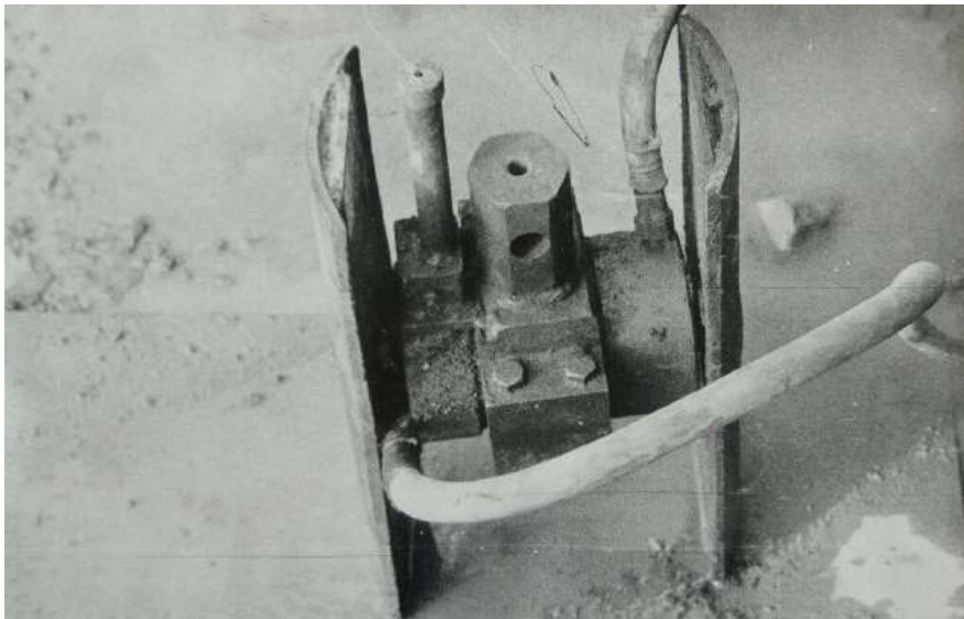
Рис.1. Лопатевий пресіометр гідравлічний ЛПГ-42 конструкції Л.С. Амаряна
